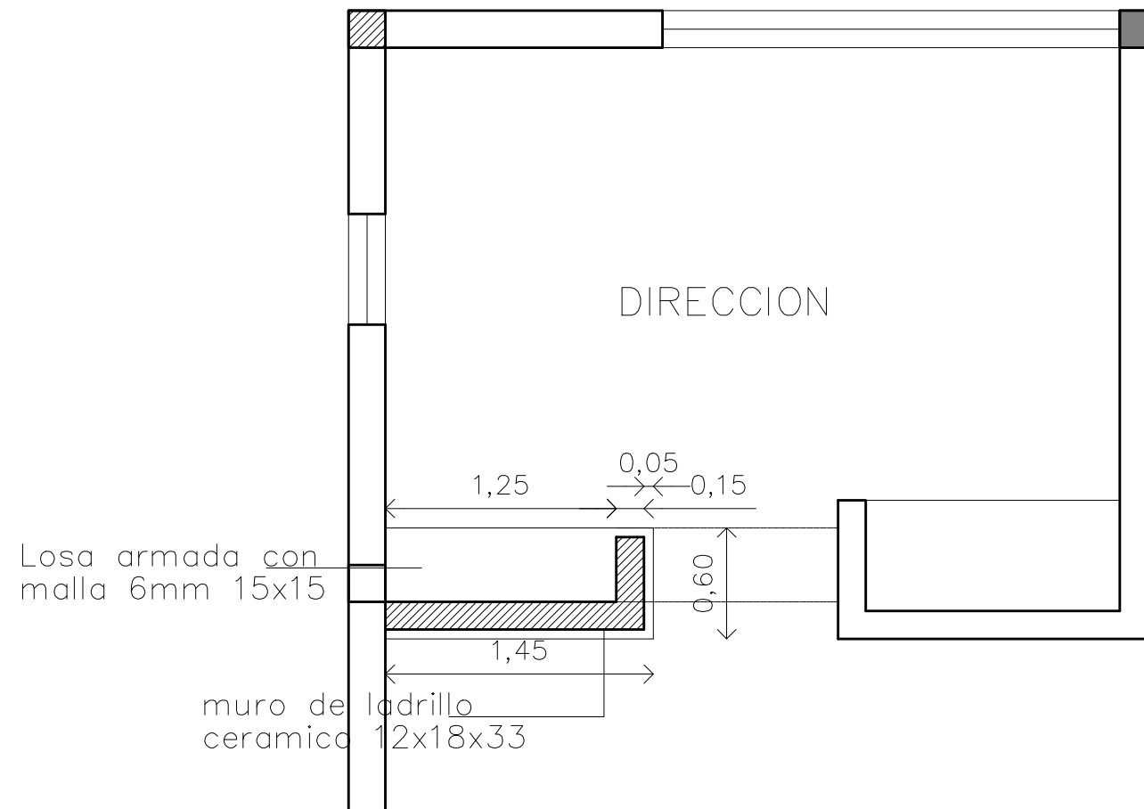
Planta
